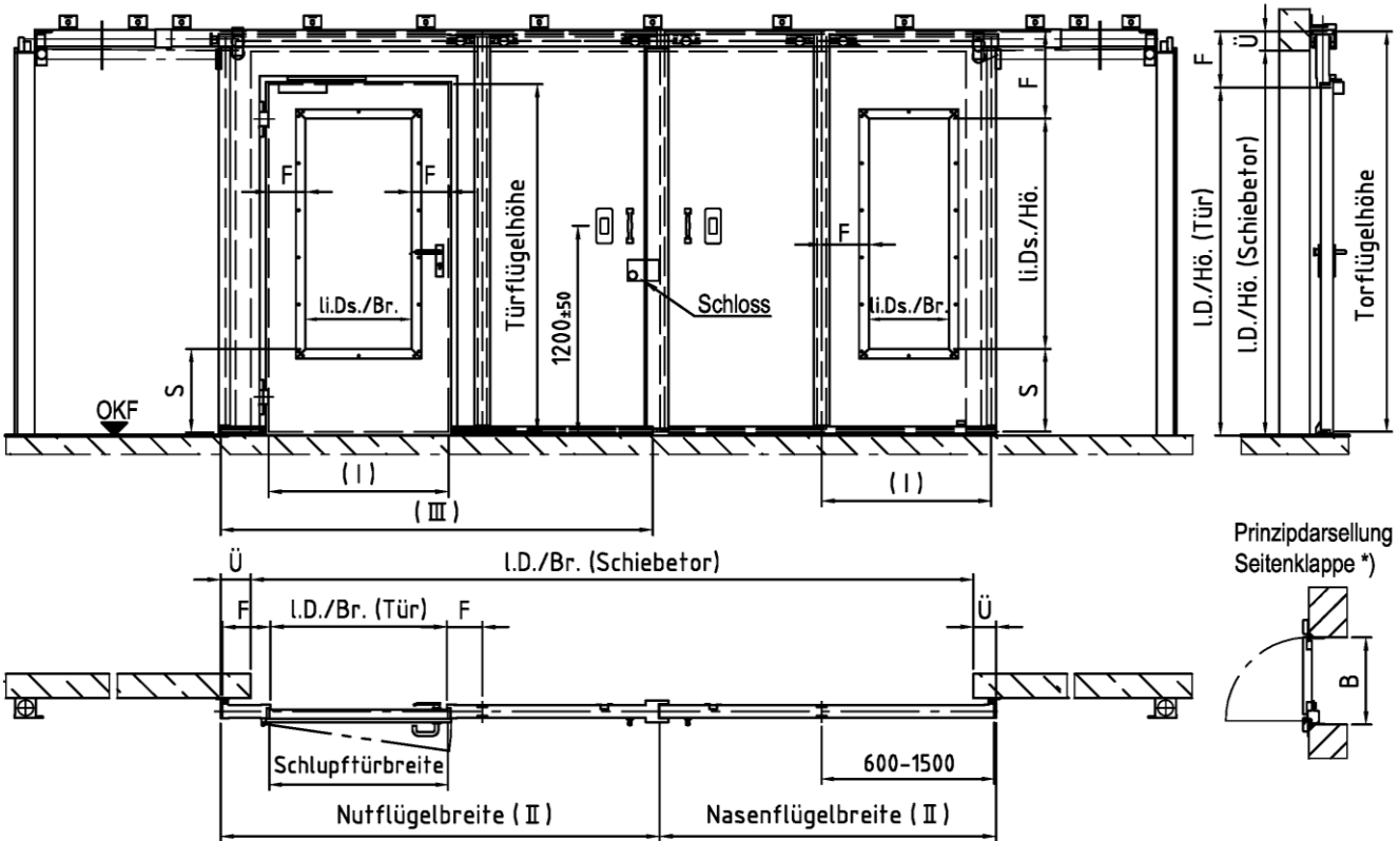
T90-2 Prinzipdarstellung *)
