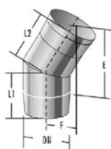
3) Bogen starr Winkel: 15°/30°/45°
