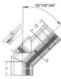
4b) Bogen starr mit RV-Deckel, druckdicht Winkel: 15°/30°/45°
