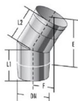
4a) Bogen starr Winkel: 15°/30°/45°
