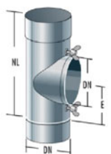
5) T-Stück mit Bolzen
