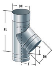
11) Feuerungsanschluss 45° mit Kondensatabtropfkante
