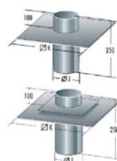
7) Dehnfugenblech nur für trockenen Betrieb
