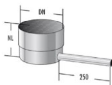
21) Kondensatschale mit Ablauf
