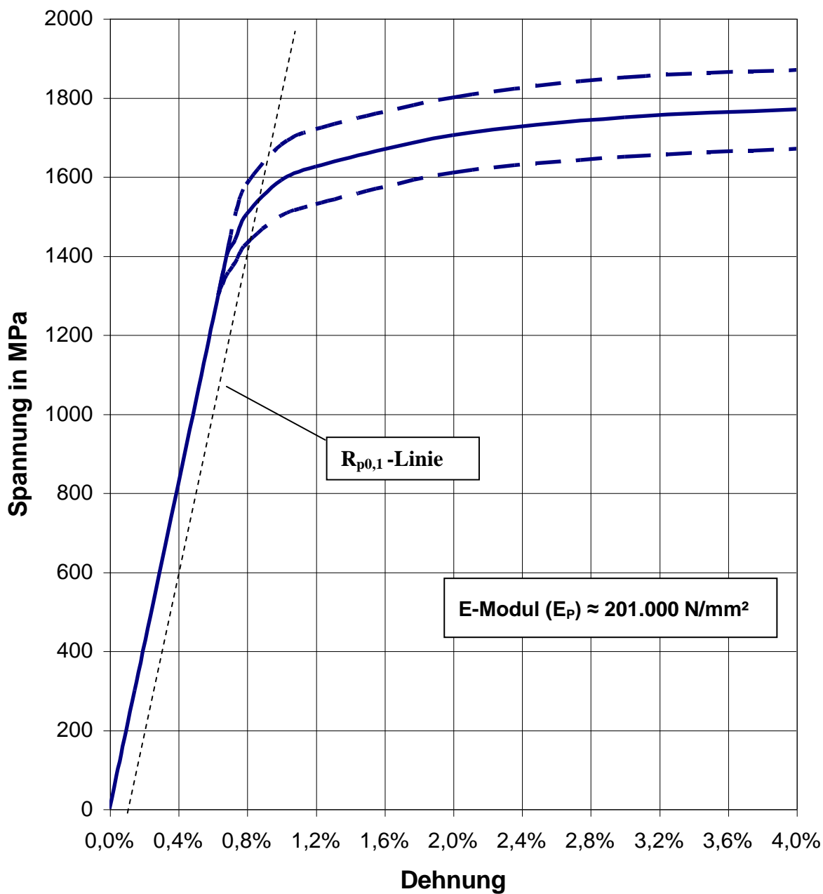
Bild 2: Spannungs-Dehnungs-Linie
