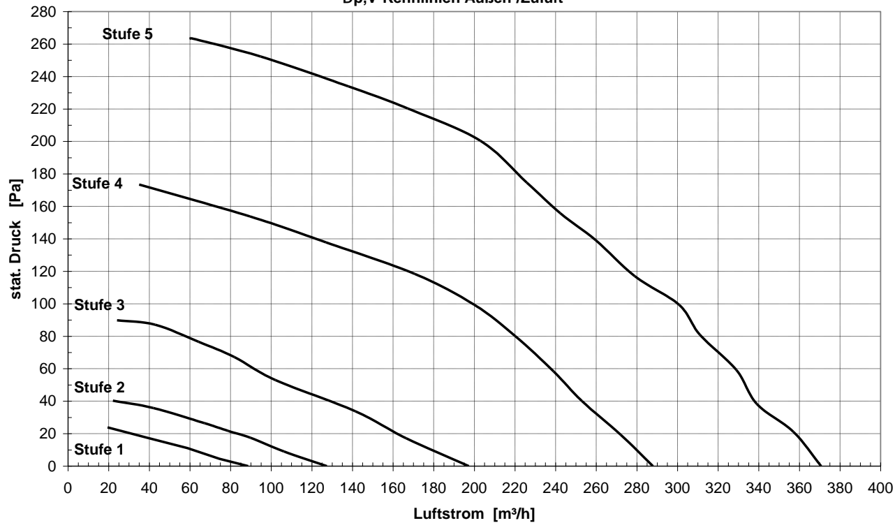
Dp,V-Kennlinien Außen-/Zuluft
