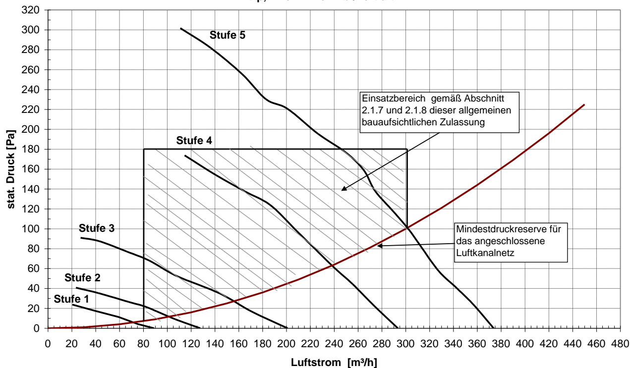
Dp,V-Kennlinien Ab-/Fortluft
