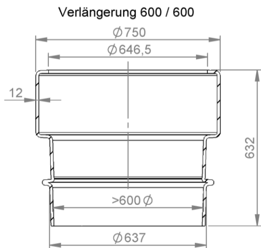
SCHNITT A-A
