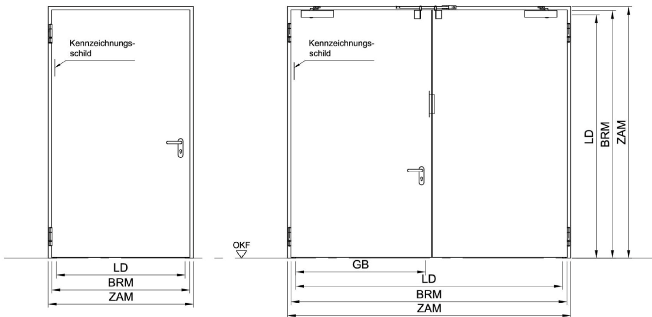
Dargestellt: Gangflügel DIN links, Gangflügel DIN rechts spiegelbildlich Maße in mm
