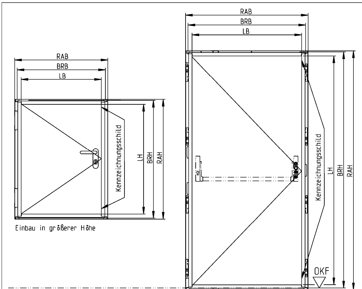
Ansicht Schließseite
