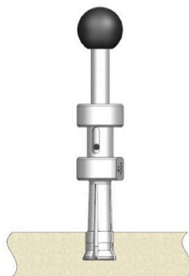
HVL (Hinterschnitt-Mindestvolumenlehre)
