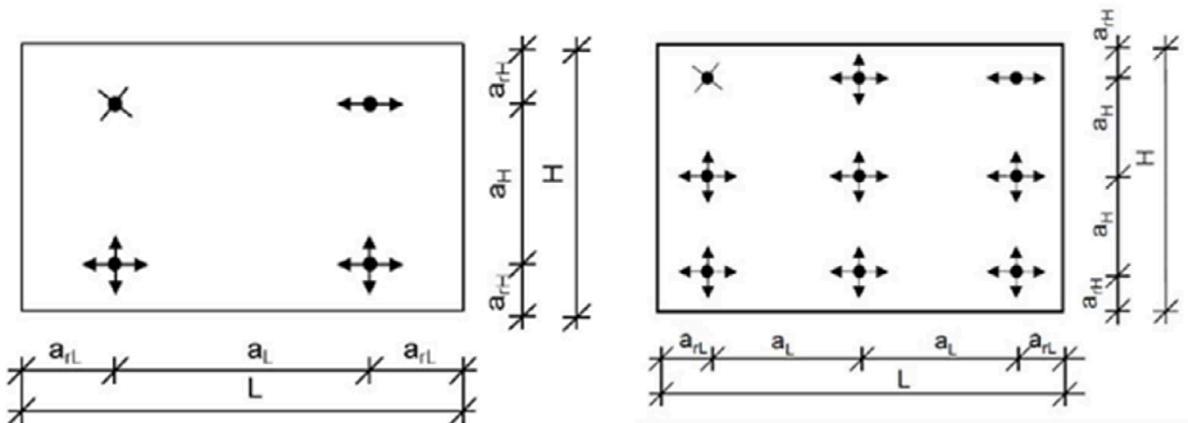
Bild B1: Definition von Rand- und Achsabstand
