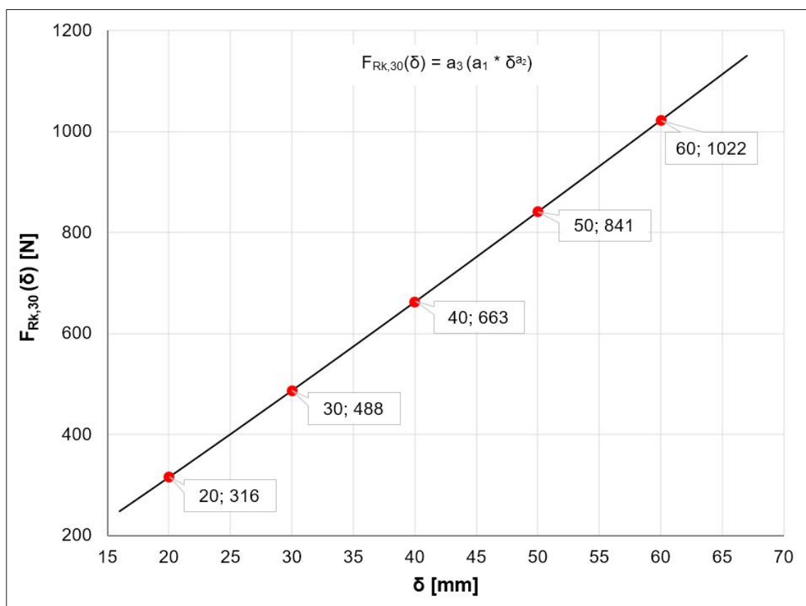
Abbildung D12: Regressionskurve gemäß Tabelle D12
