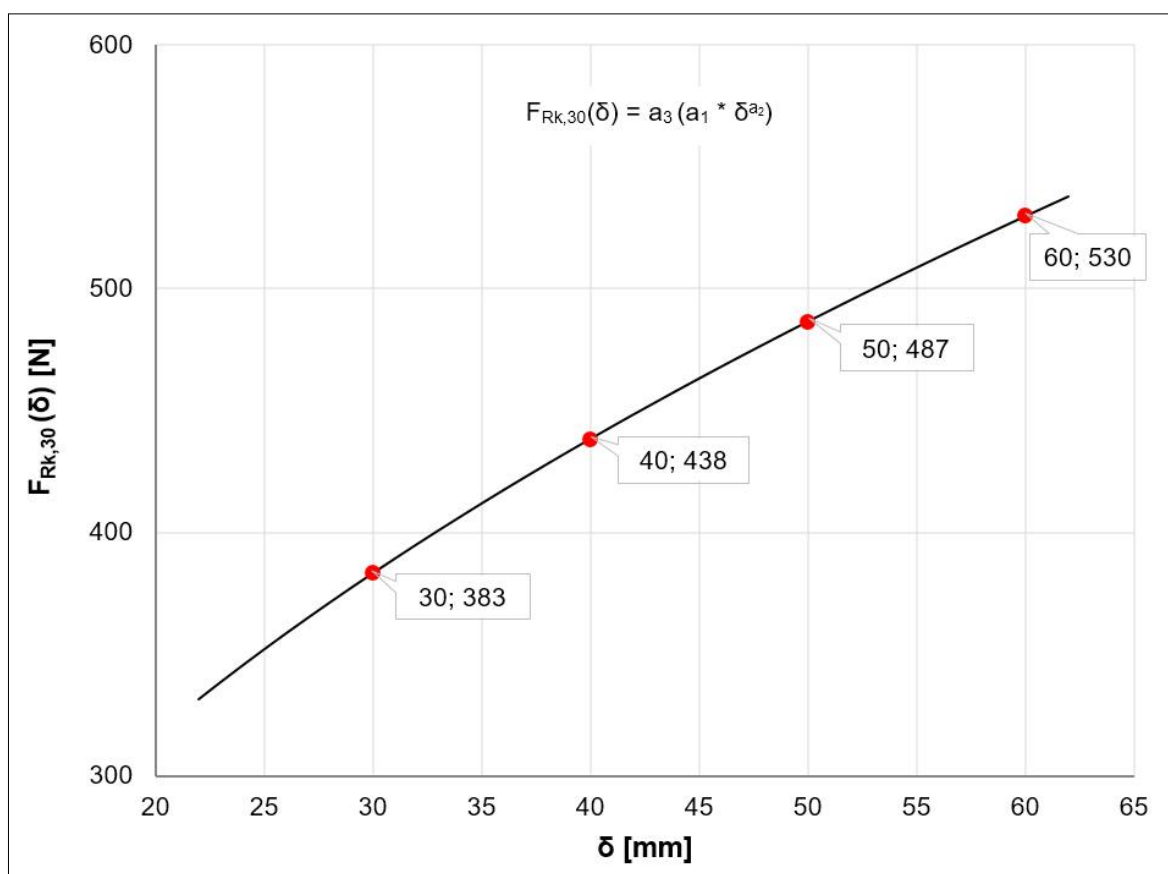
Abbildung D10: Regressionskurve gemäß Tabelle D10
