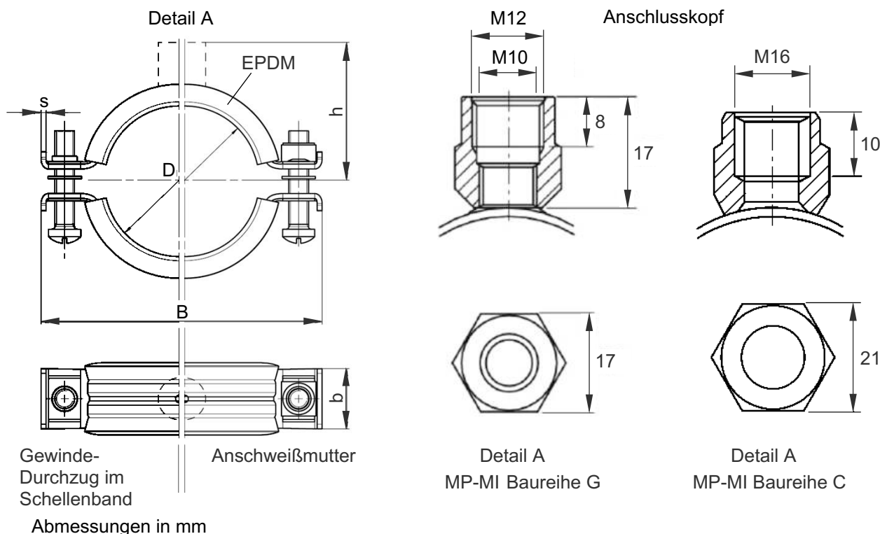
Abbildung A1: Geometrie und Abmessungen der Massivrohrschellen MP-MI, Baureihe G mit Anschlusskopf M10/M12, Baureihe C mit Anschlusskopf M16
