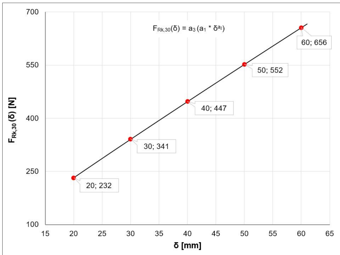
Abbildung D4: Regressionskurve gemäß Tabelle D4
