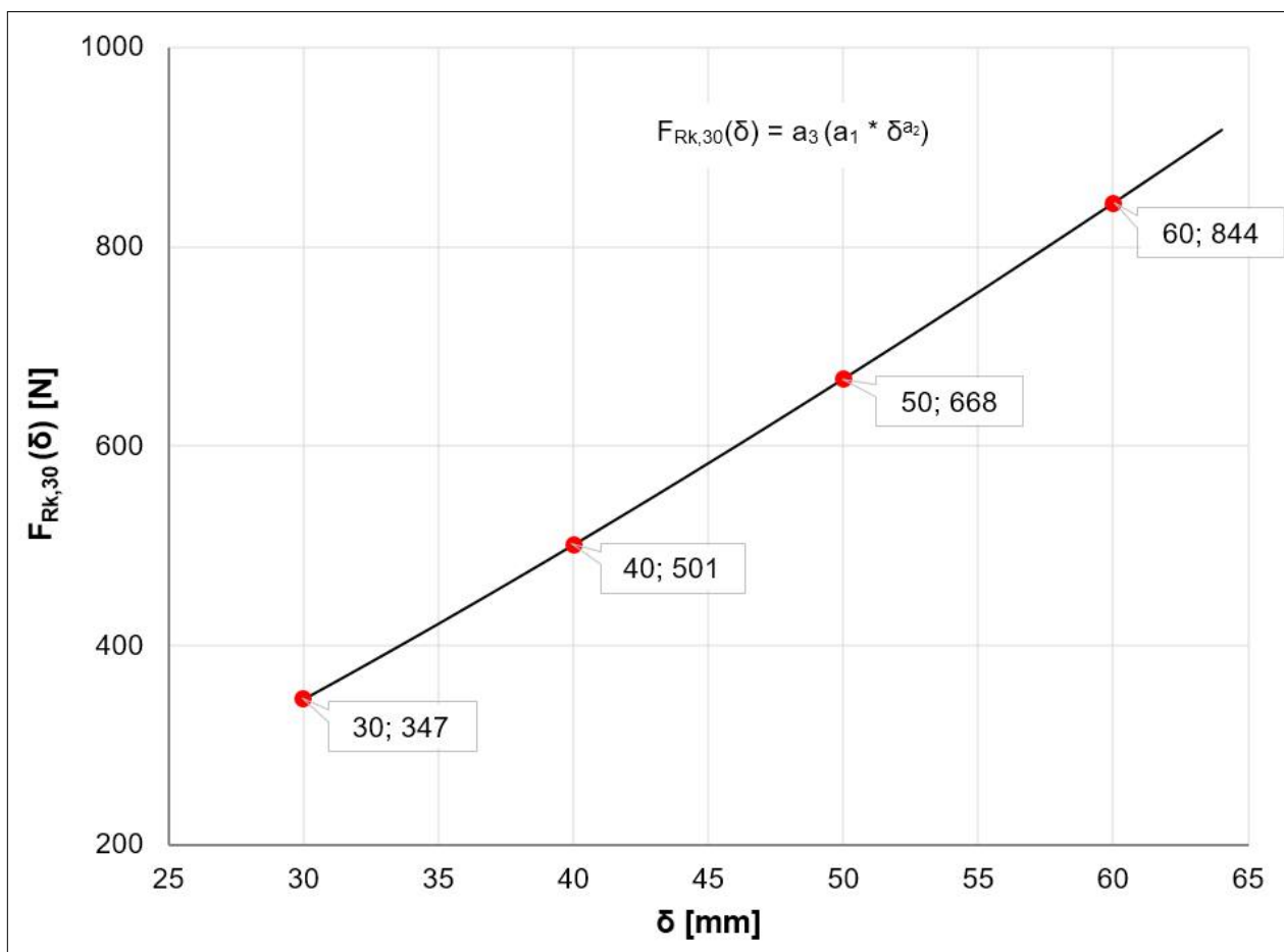
Abbildung D8: Regressionskurve gemäß Tabelle D8 Bezeichnungen siehe Anhang D2
