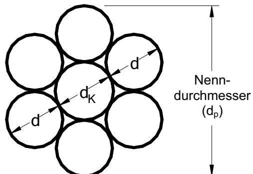
Bild 1: Darstellung des Spannstahlлитzen-Querschnitts
