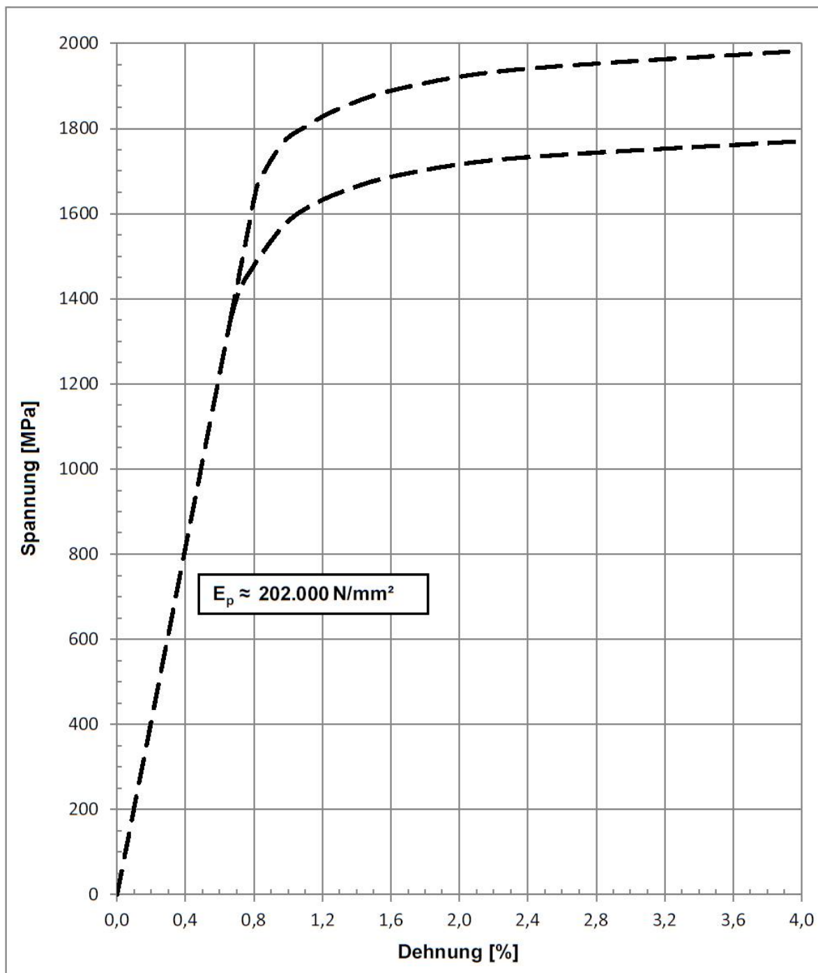
Bild 2: Prinzipieller Spannung-Dehnungs-Verlauf
