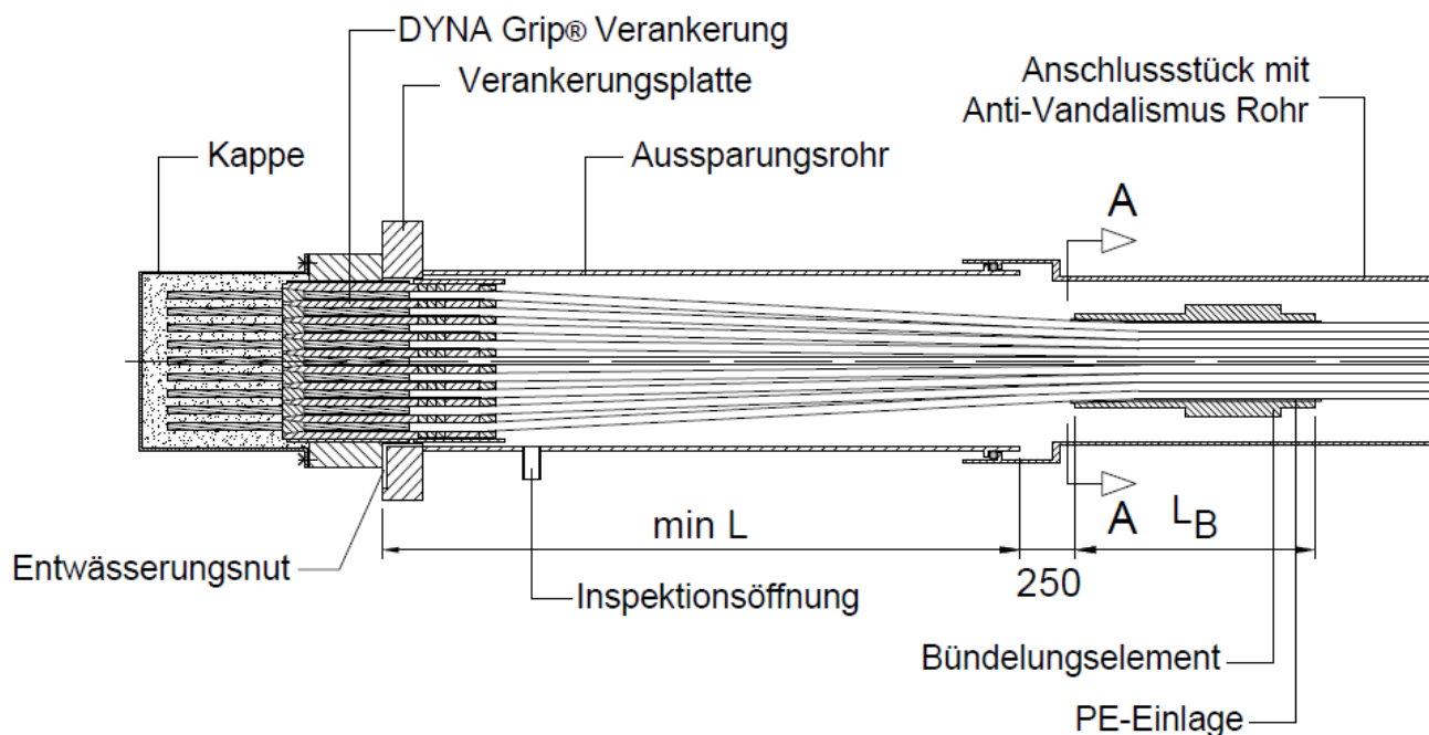
Schnitt A-A Typ 12
