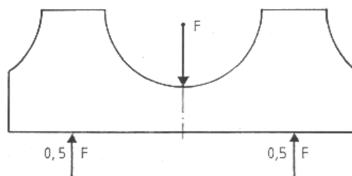
Bild 1: Belastungsanordnung Biegeversuch
