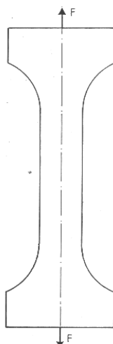
Bild 2: Belastungsanordnung Zugversuch
