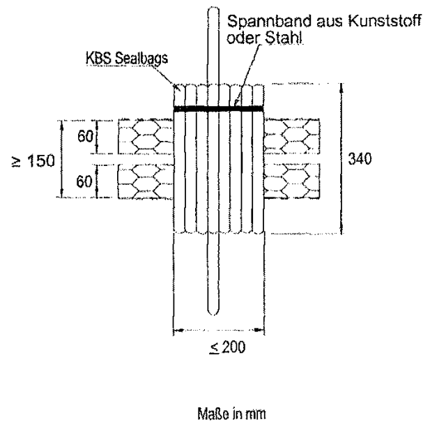
Schnitt D - D Deckeneinbau
