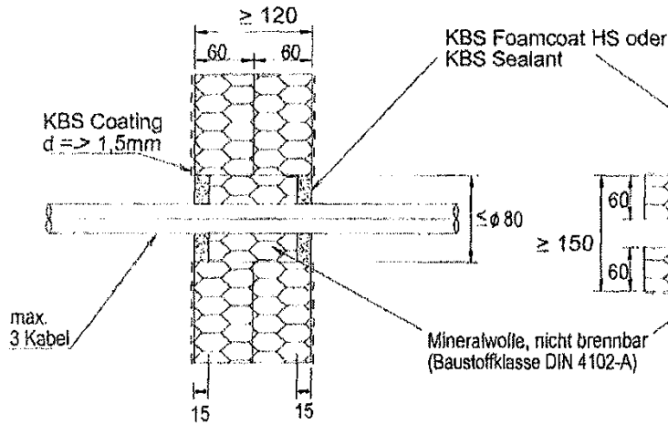
Schnitt E - E Wandeinbau
