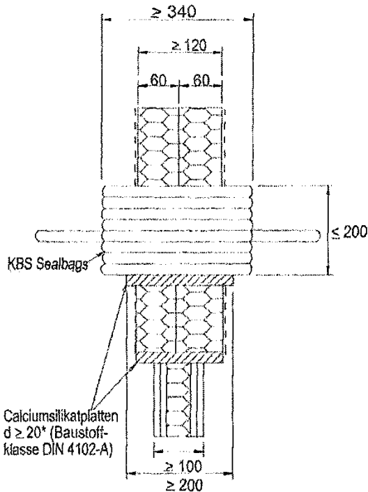
Schnitt D - D Wandeinbau
