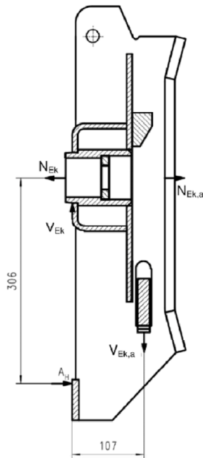
Bild 13: PERI Kletterschuh I ACS
