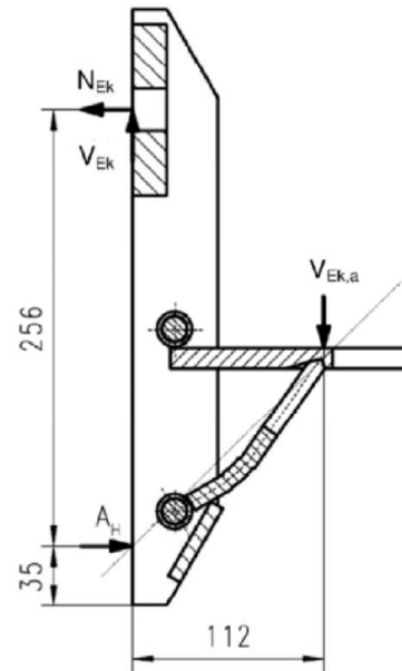
Bild 9: PERI Klappkonsole 25
