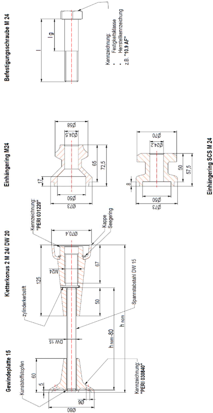
Bild 5: Einzelteile, Abmessungen Kletterkonus-2 M 24/DW 15
