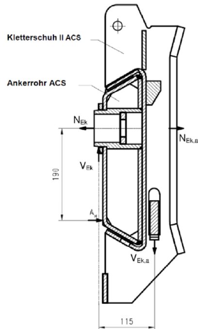
Bild 14b: PERI Kletterschuh II ACS
