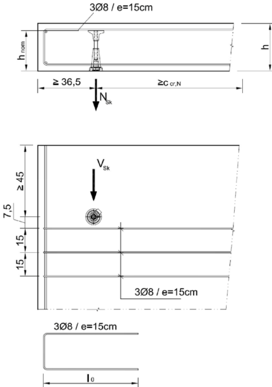
Bild 19: Randeffassbewehrung unterhalb des Konus (entsprechend Querkraftfrichtung) 3 Ø8mm mit e = 15 cm, die mit der Wandbewehrung voll zu übergreifen sind.
