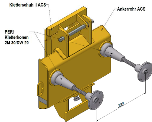
Bild 14a: PERI Kletterschuh II ACS (Isometrie)
