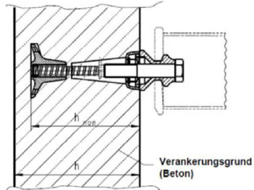
Bild 1: PERI Kletterkonus-2 M 24/DW 15 mit PERI Einhänger M24
