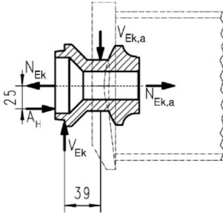
Bild 12: PERI Einhängerling M30
