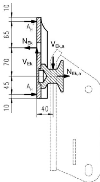
Bild 10: PERI Aufhängeschuh FB
