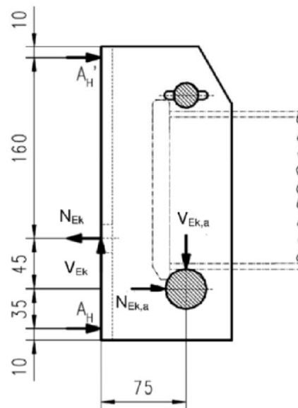
Bild 11: PERI Wandgerüstschuh WGS
