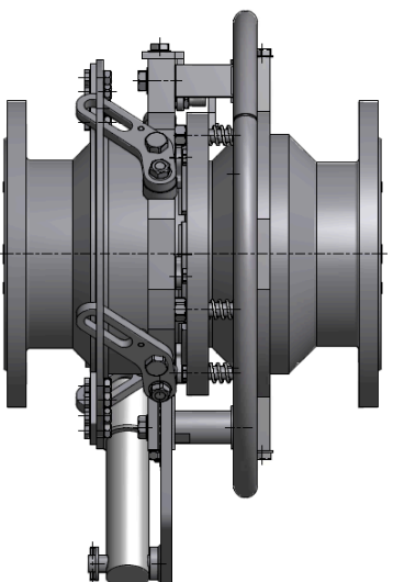
NTS-H Auslösung: Hydraulik
