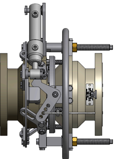
NTS-SZ-H Auslösung: Hydraulik + Seil
