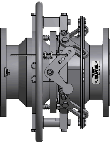
NTS-SZ Auslösung: Seilzug
