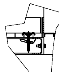
Detail B Gitterrostklemme
