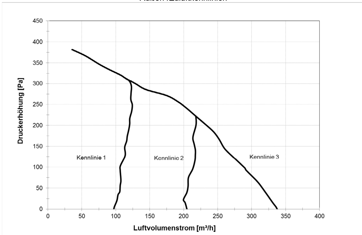
Außen-/Zuluftkennlinien
