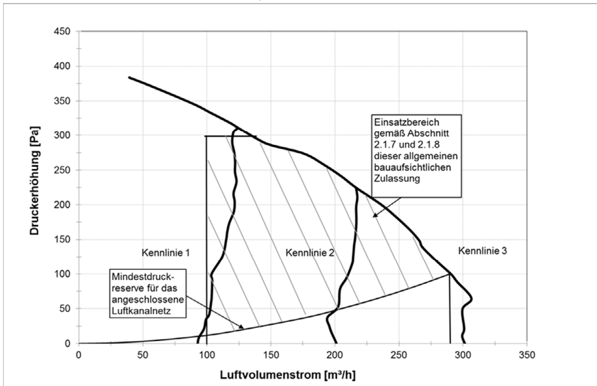
Ab-/Fortluftkennlinien
