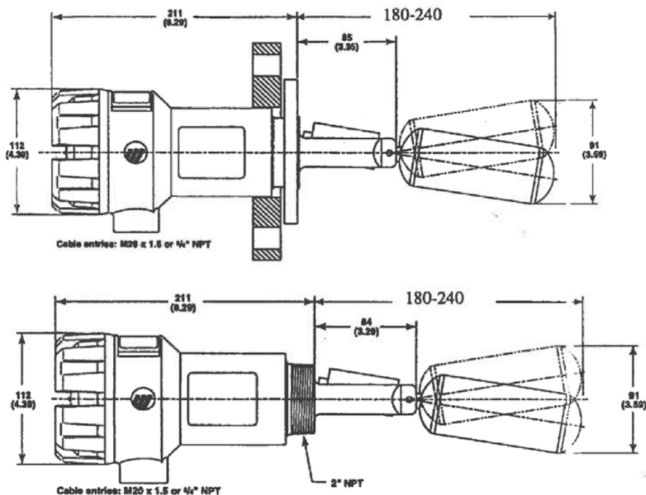
Schema für den Aufbau von Überfüllsicherungen
