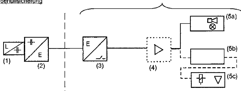
Schema der Überfüllsicherung
