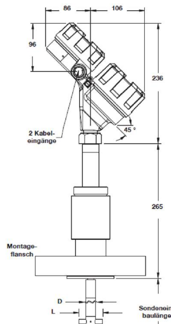
Modell 7yJ mit Flanschanschluss
