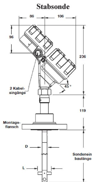
Modell 7yG mit Flanschanschluss
