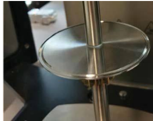
Abb. A 4.1: Versuchsaufbau, Rheometer
