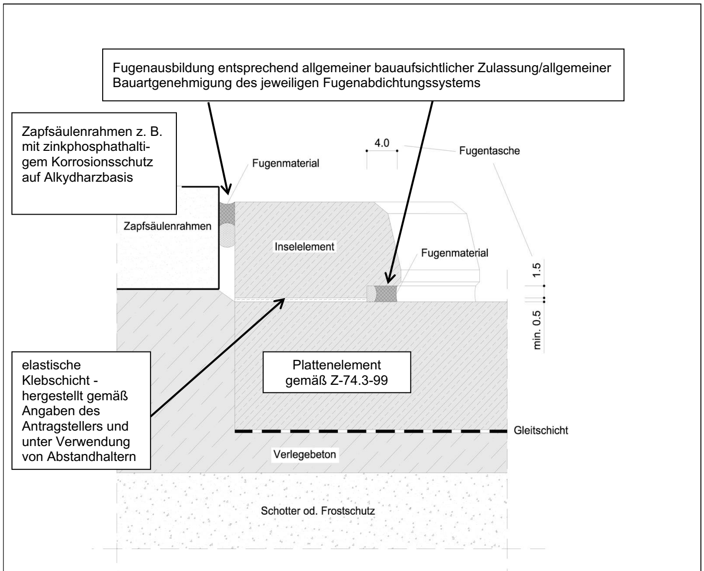
Abbildung 1: Beispiel Anschluss Inselement an anschließende Konstruktion
