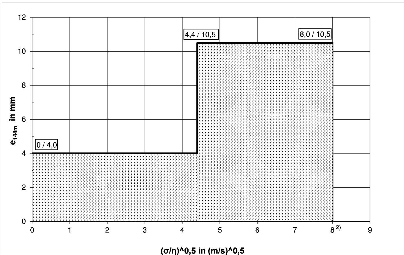
Abbildung 1: Eindringverhalten (mittlere Eindringtiefe e_{144m} nicht betonangreifender Flüssigkeiten) 1,2 , aufgrund der jeweiligen dynamischen Viskosität \eta und Oberflächenspannung \sigma
