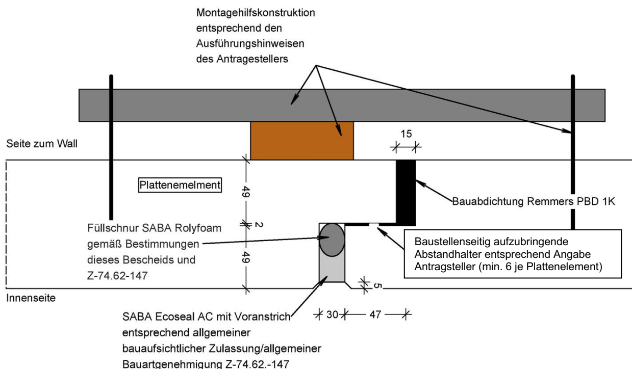
Abbildung 2: Montagehilfsmittel im Plattenstoß
