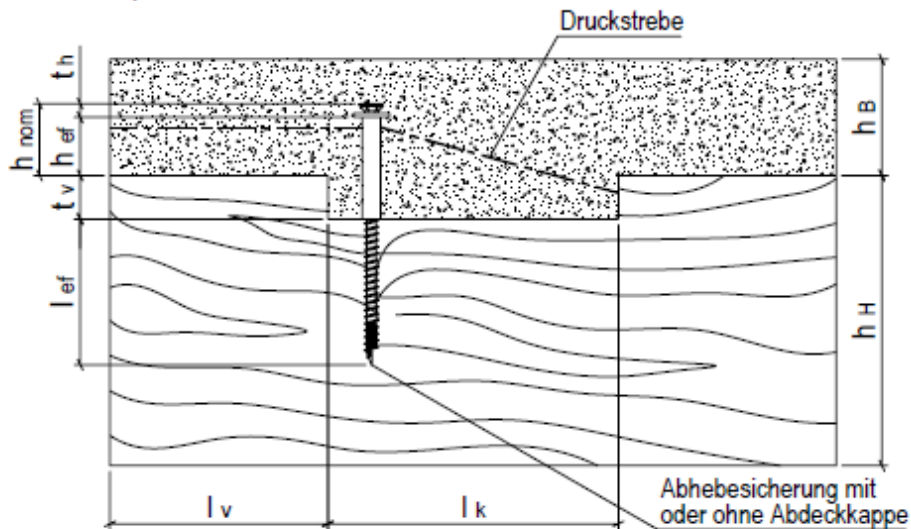
Abbildung 1: Prinzipskizze der Wirkungweise von Reisser Schrauben als Abhebesicherung bei tragenden Holz-Beton-Verbundkonstruktionen mit Kerven als Schubverbund für den Einsatz in Holz-Beton-Verbundbauteilen - Abhebesicherung in der Kerbe
