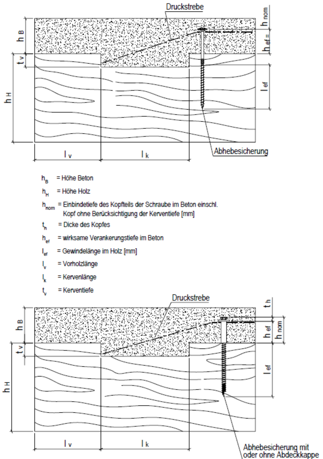
Abbildung 2: Prinzipskizze der Wirkungsweise von Reisser Schrauben als Abhebesicherung bei tragenden Holz-Beton-Verbundkonstruktionen mit Kerven als Schubverbund für den Einsatz in Holz-Beton-Verbundbauteilen - Abhebesicherung außerhalb der Kerve
