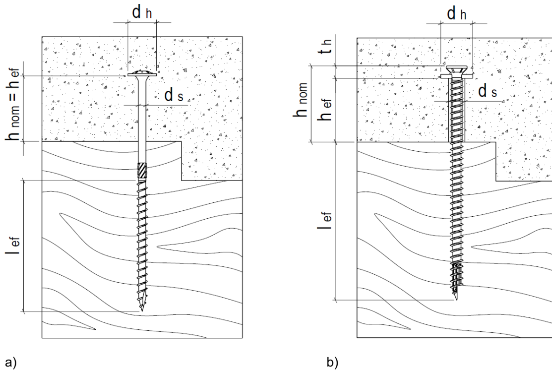
Abbildung 5: Definition der wirksamen Verankerungstiefe
