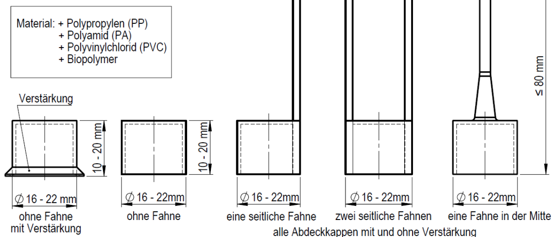
Abbildung 4: Abdeckkappen, verschiedene Varianten
