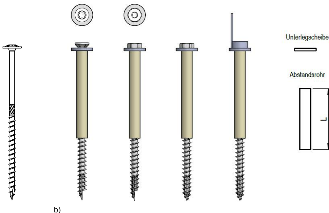
Abbildung 3: Reisser Schrauben für den Einsatz in Holz-Beton-Verbundbauteilen
