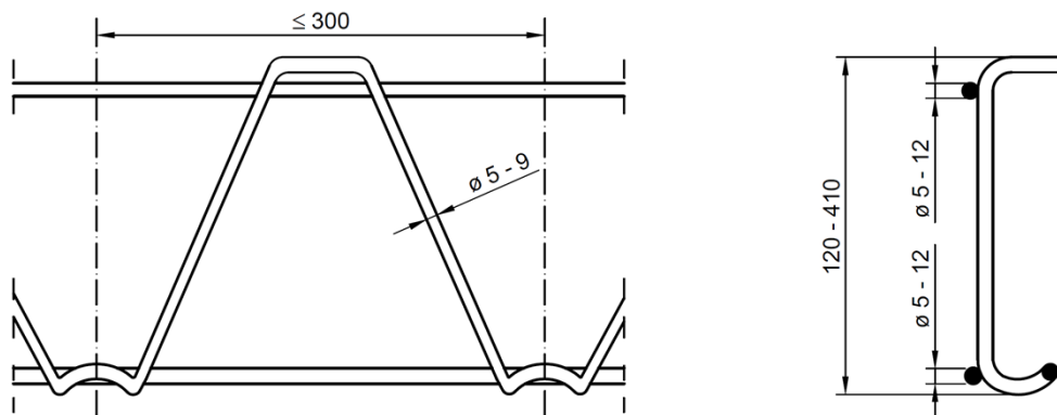
Bild 5: Filigran-SWE-Gitterträger
