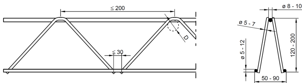
Bild 1: Filigran-D-Gitterträger
