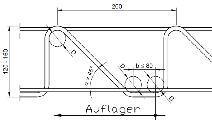
Bild 7: Filigran-EQ-Gitterträger
