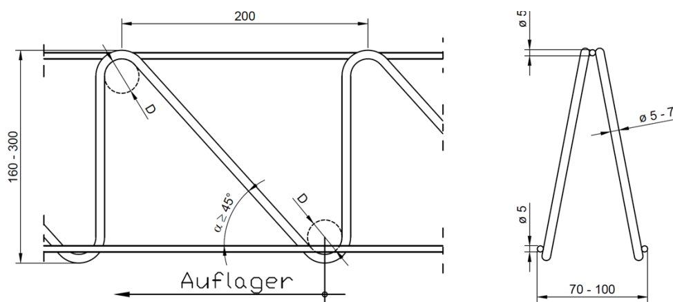
Bild 7: Filigran-EQ-Gitterträger
