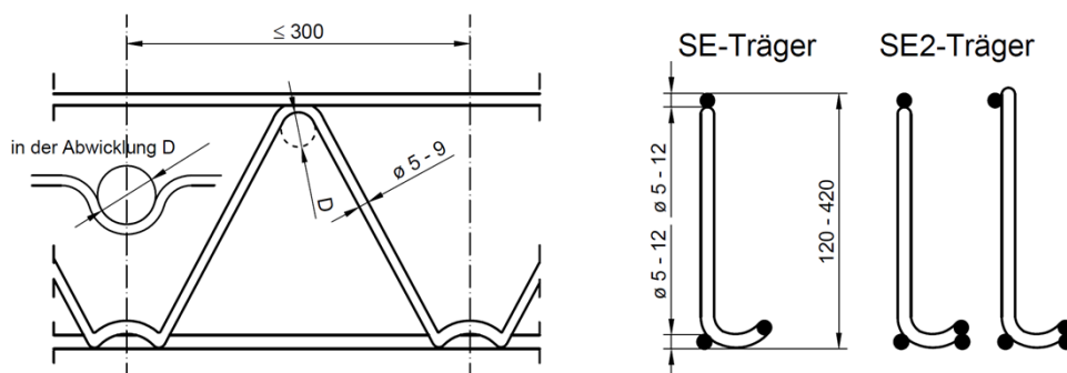
Bild 4: Filigran-SE/SE2-Gitterträger
