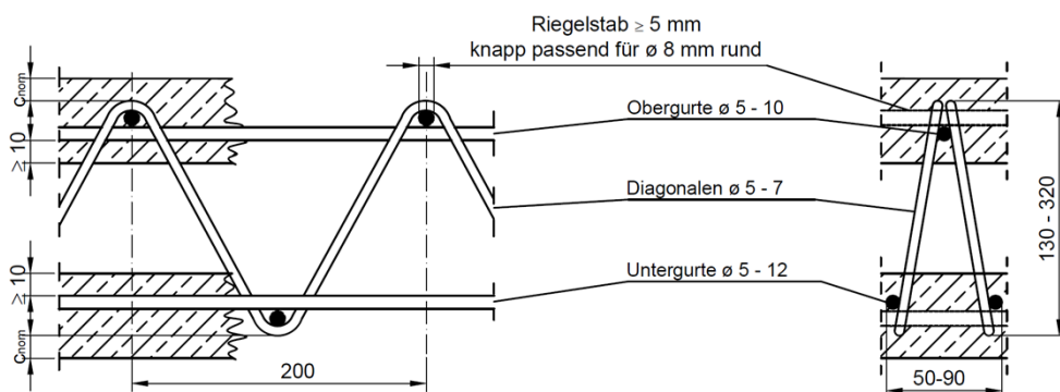
Bild 4: Filigran-SE/SE2-Gitterträger
