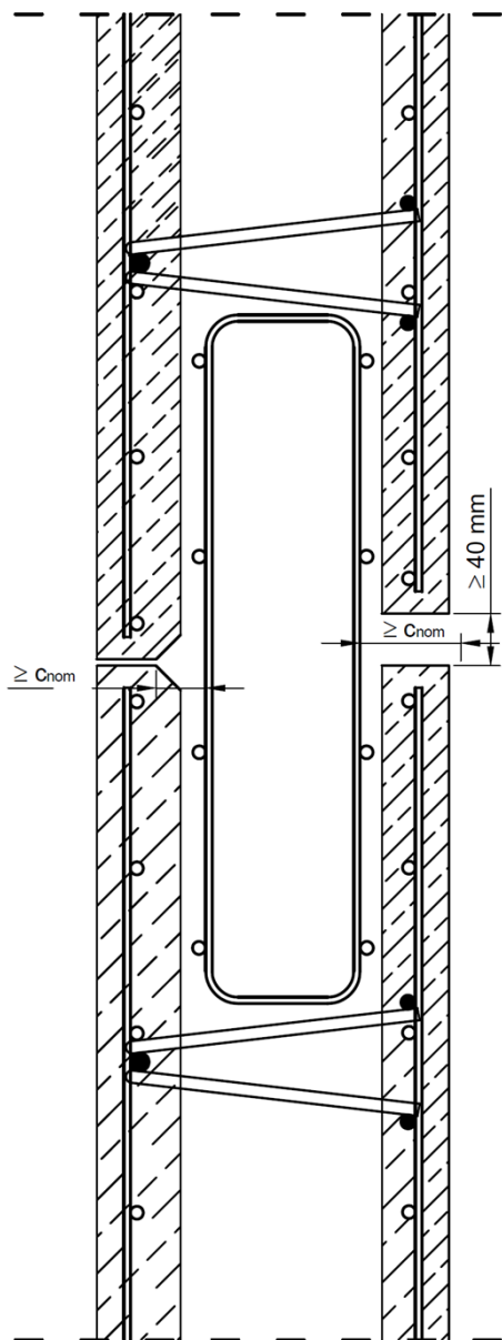
Bild 20: Fugenausbildung
