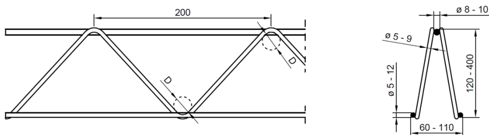
Bild 2: Filigran-E-Gitterträger
